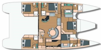
Plan d'aménagement proposé - 4 Cabines + quart équipage
